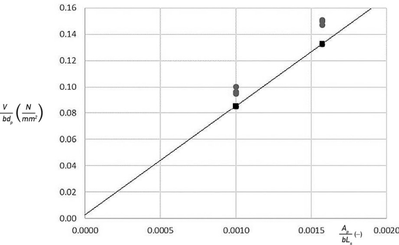
Υπολογισμός των συντελεστών m - k από τα πειραματικά αποτελέσματα για το SYMDECK 100.
