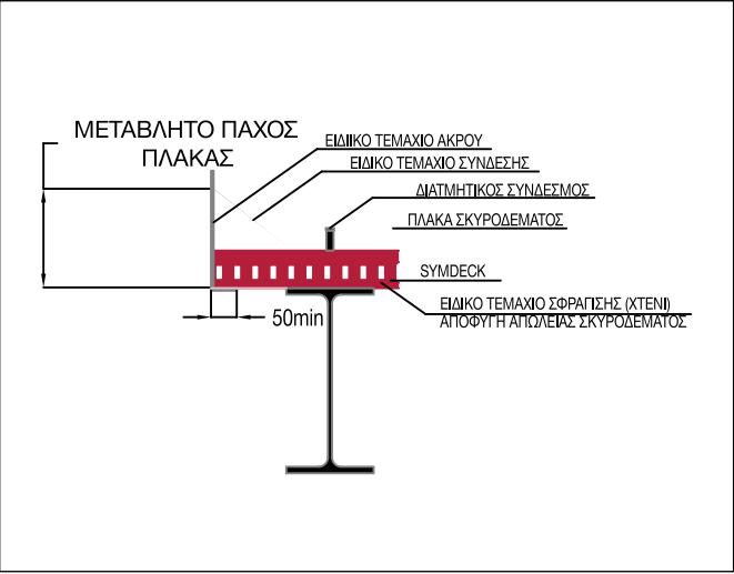
ΛΕΠΤΟΜΕΡΕΙΑ ΤΕΛΟΥΣ ΠΛΑΚΑΣ ΜΕ ΠΡΟΒΟΛΟ
