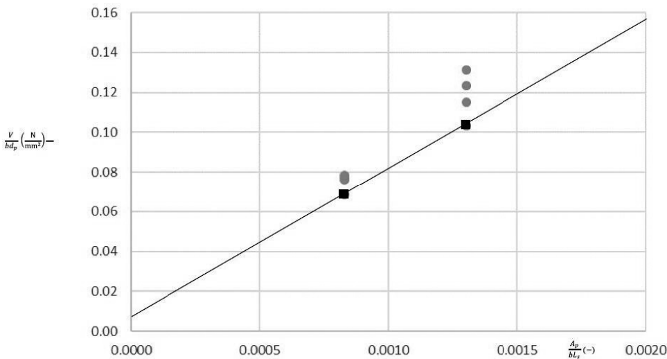
Υπολογισμός των συντελεστών m - k από τα πειραματικά αποτελέσματα για το SYMDECK 50.
