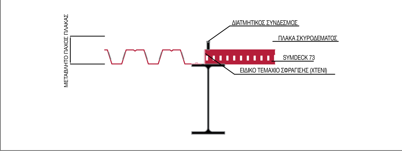
ΛΕΠΤΟΜΕΡΕΙΑ ΕΝΔΙΑΜΕΣΗΣ ΔΟΚΟΥ ΜΕ ΑΛΛΑΓΗ ΔΙΕΥΘΥΝΣΗΣ ΣΤΡΩΜΑΤΟΣ
