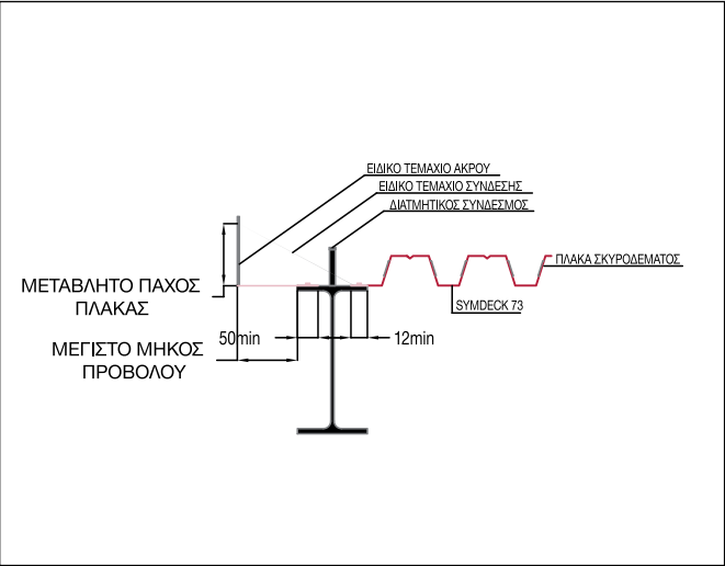
ΛΕΠΤΟΜΕΡΕΙΑ ΑΚΡΟΥ ΜΕ ΠΡΟΒΟΛΟ
