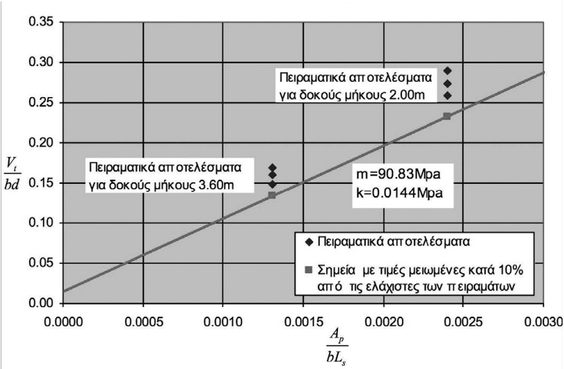
Υπολογισμός των συντελεστών m - k από τα πειραματικά αποτελέσματα για το SYMDECK 73.
