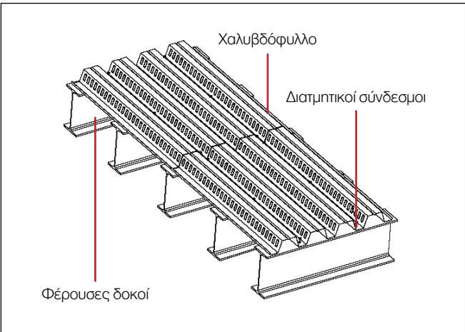
Σχήμα 1: Τυπική διάταξη υποδομής σύμμικτης πλάκας.
