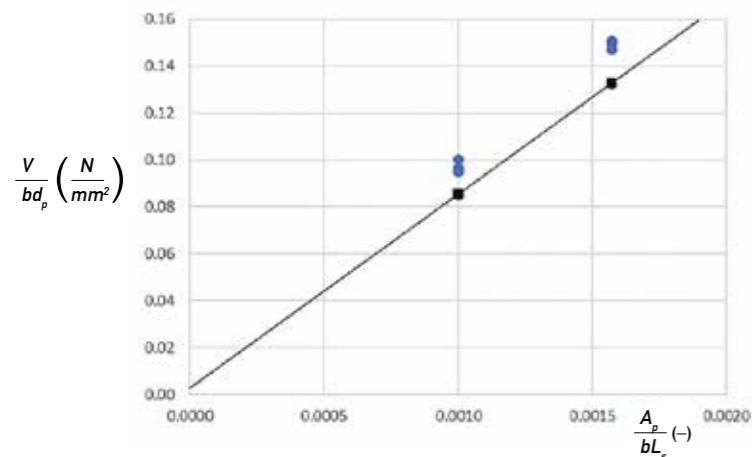
Σχήμα 2: Υπολογισμός των συντελεστών m-k από τα πειραματικά αποτελέσματα για το SYMDECK 100.
