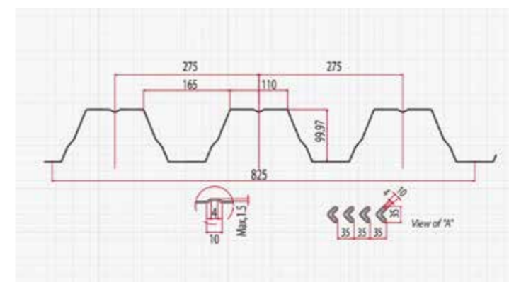
Σχήμα 1: Γεωμετρία του τραπεζοειδούς χαλυβδόφυλλου SYMDECK 100.
