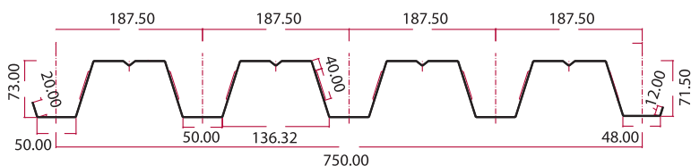
Σχήμα 3: Γεωμετρία του τραπεζοειδούς χαλυβδόφυλλου SYMDECK 73.
