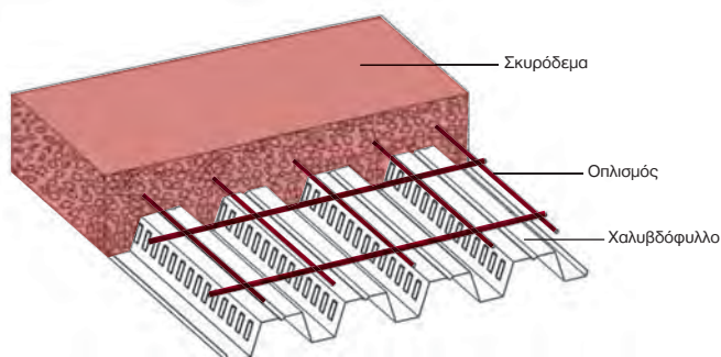
Σχήμα 2: Διαμόρφωση της σύμμικτης πλάκας.
