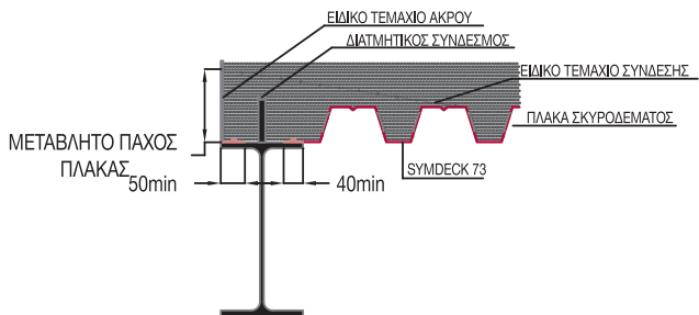
ΛΕΠΤΟΜΕΡΕΙΑ ΑΚΡΟΥ
