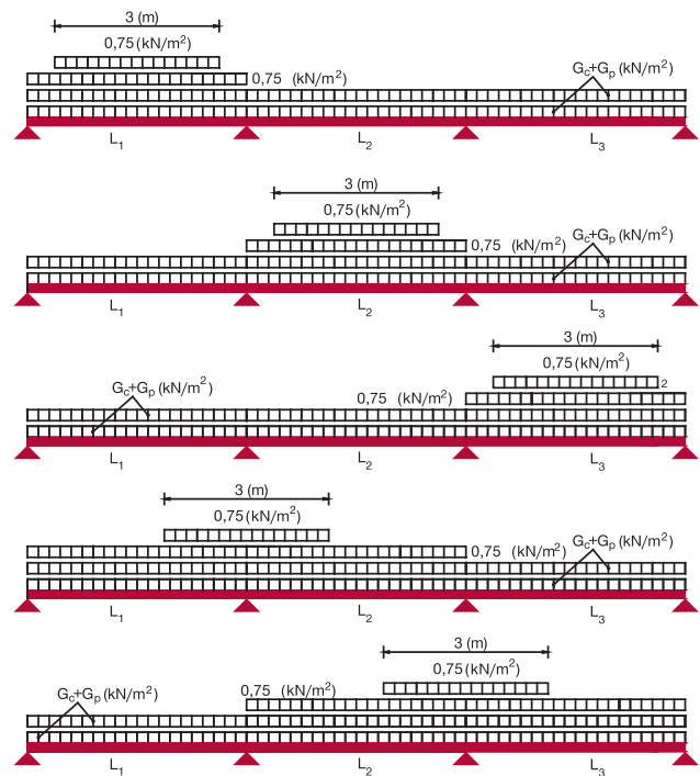
Σχήμα 10: Συνδυασμοί φορτίσεων σταδιακής διάστρωσης.
